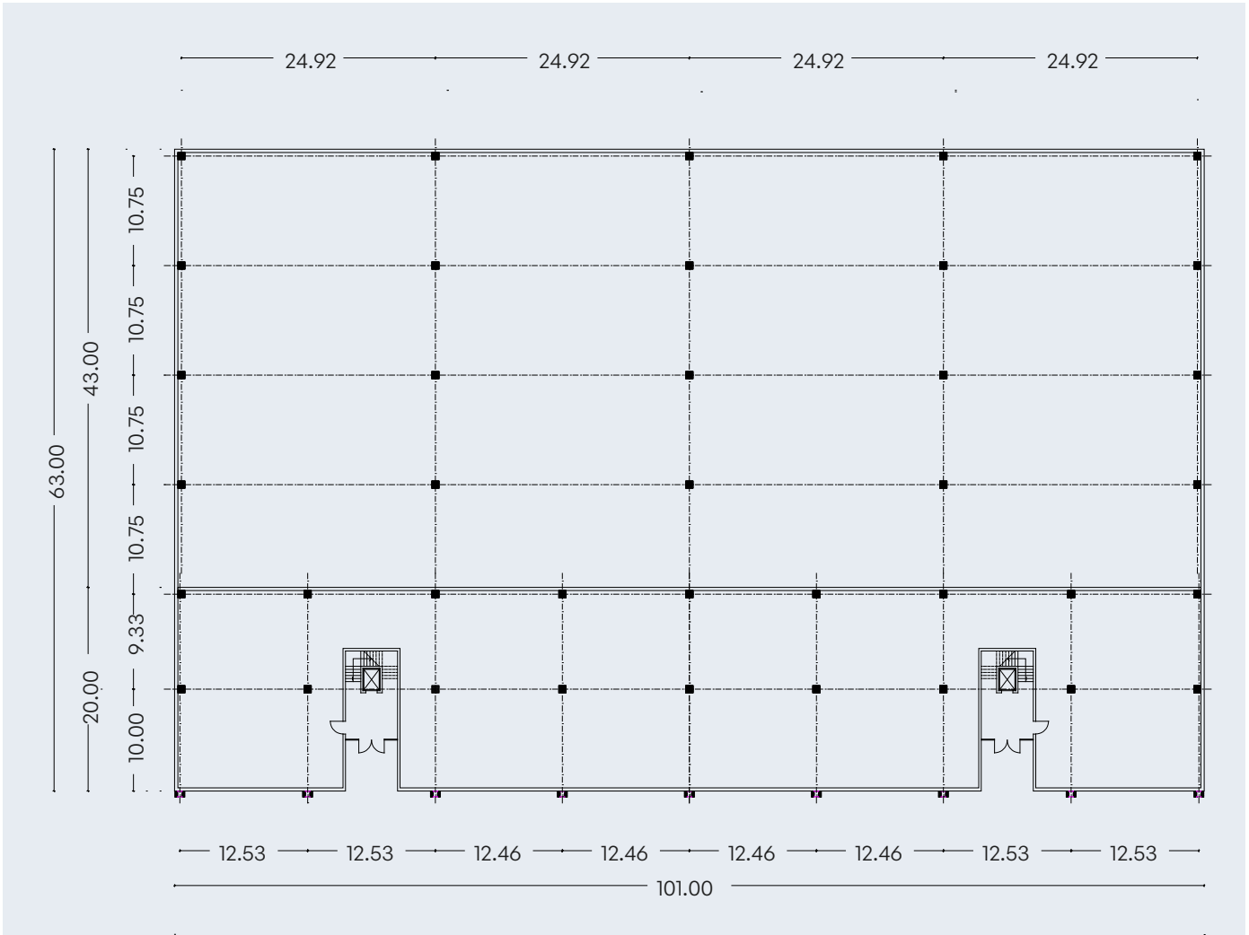
SCHEMA PILASTRATURA
